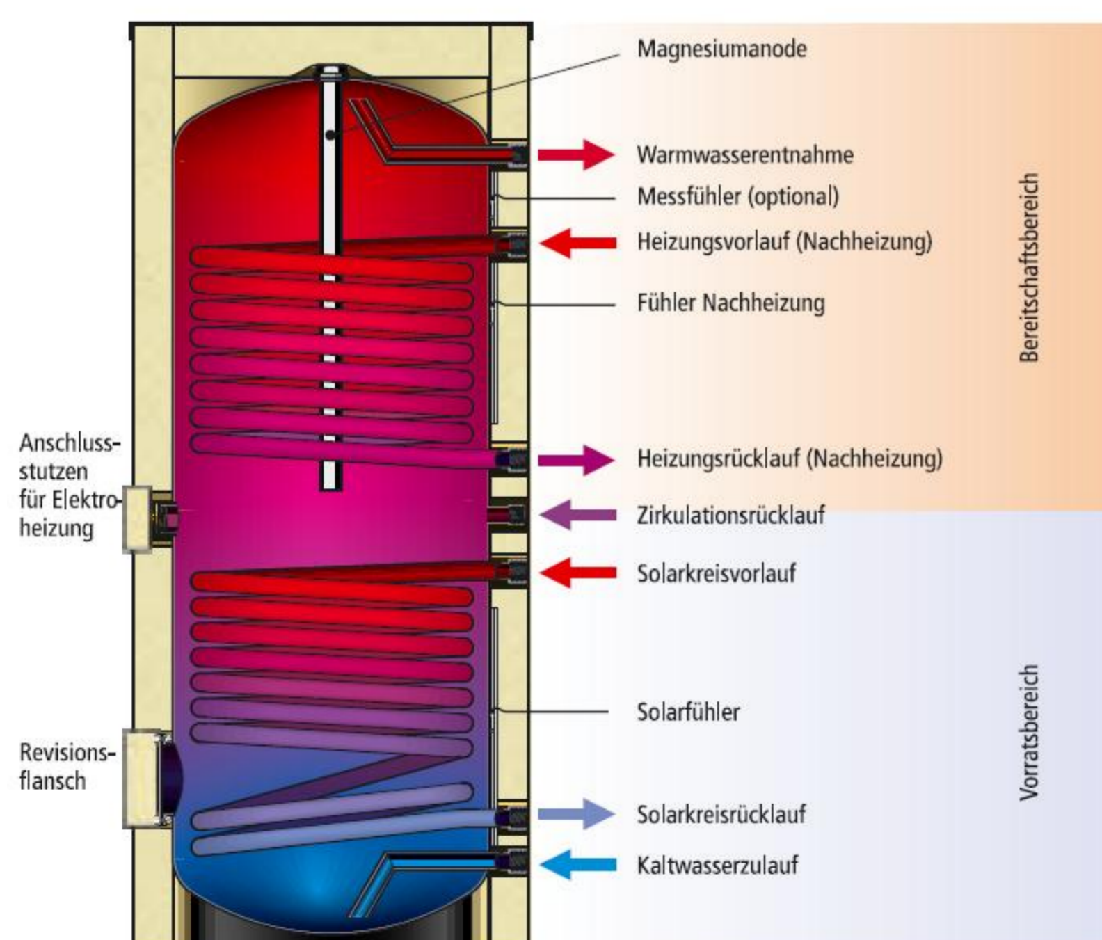
Solar-Wärmespeicher – Quelle: DGS
